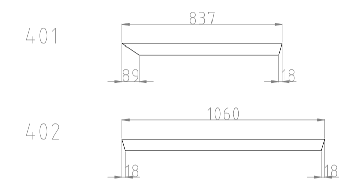
LISTE (4XX) U GALVA 60x160 EP 4
