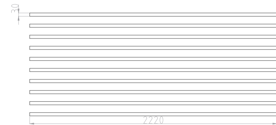
JOINTS PLATS
